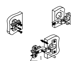
1 Регулировка створки по глубине
