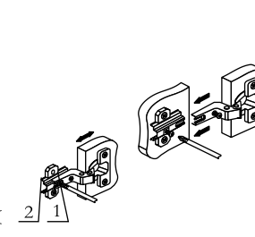
1 Регулировка створки по ширине
